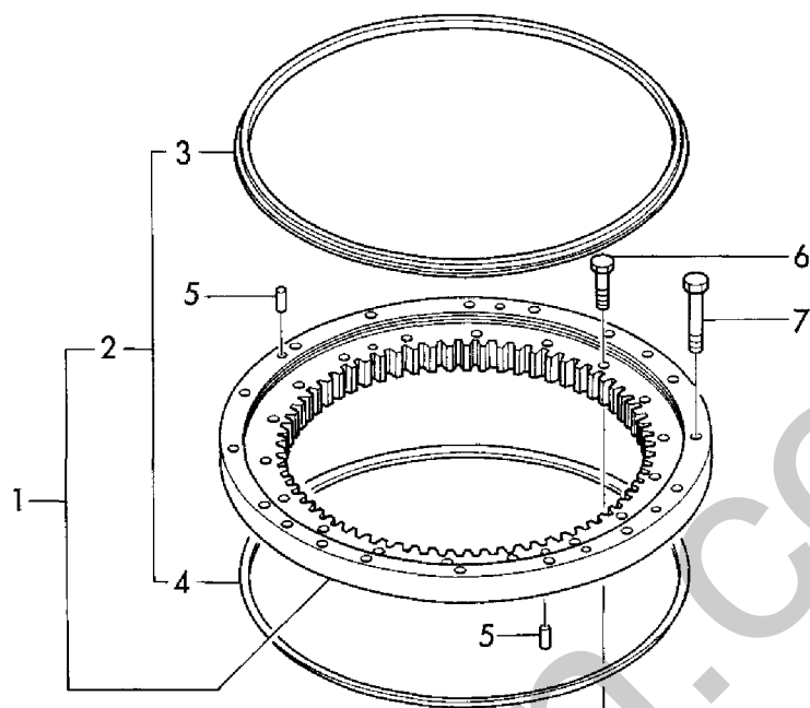
Fig. 22 旋回ベアリング TURNING BEARING
