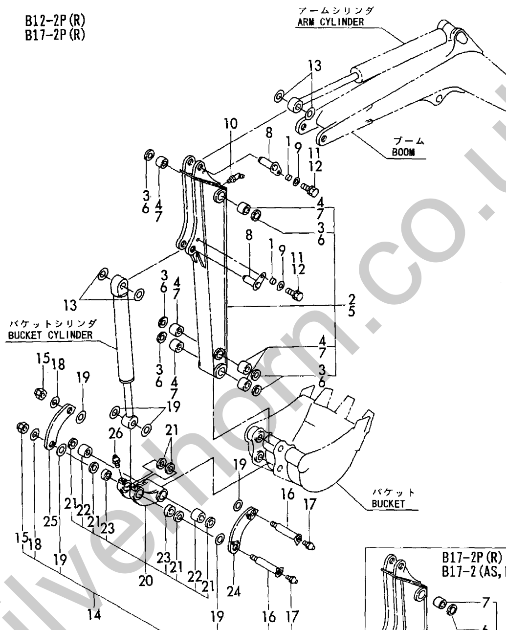
Fig. 58 アーム&バケットリンク (B12/17-2) ARM & BUCKET LINK (B12/17-2)
