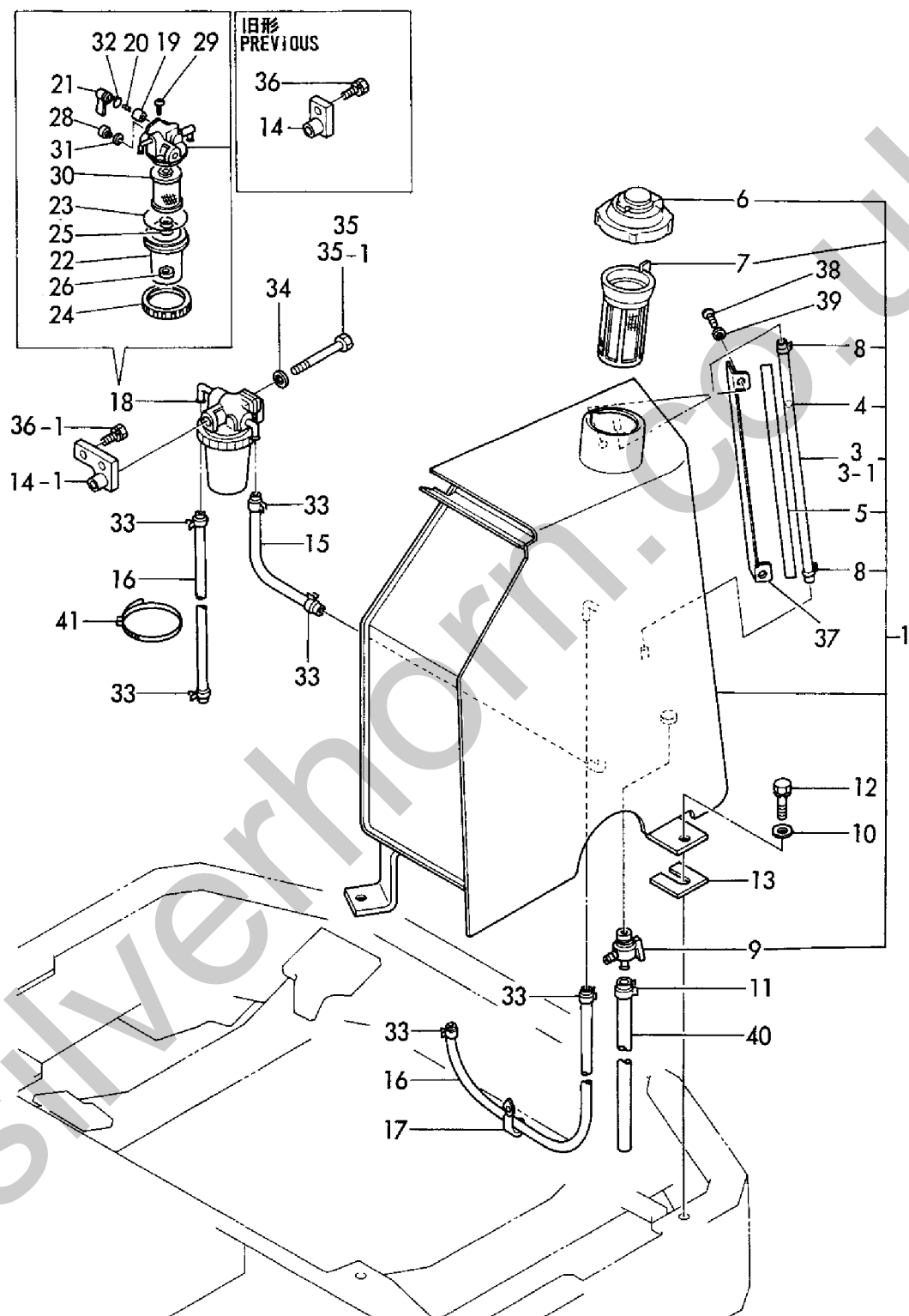
Fig. 8 燃料タンク&燃料パイプ FUEL TANK & FUEL PIPE
