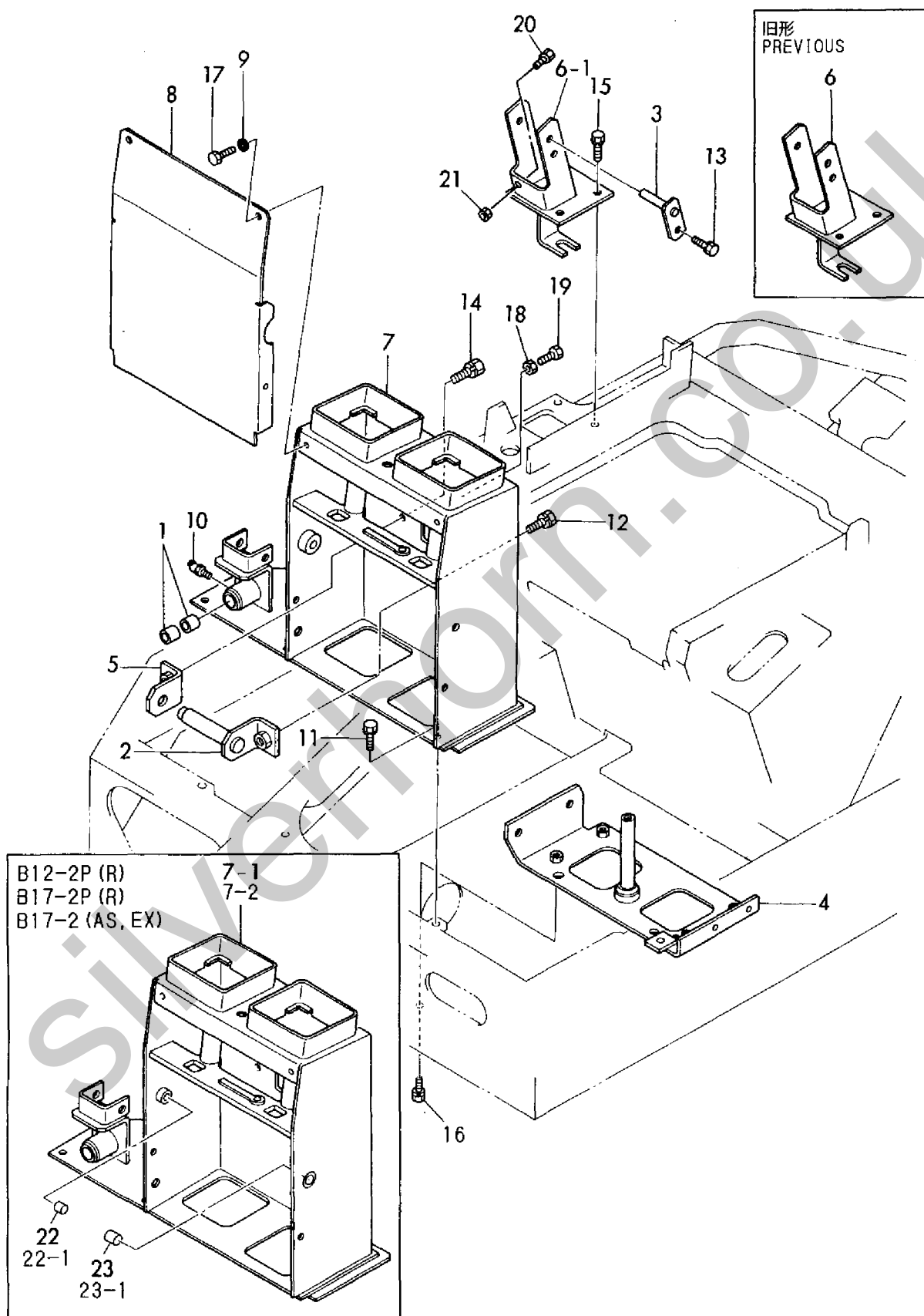
Fig. 15 リンク台 LINK STAND
