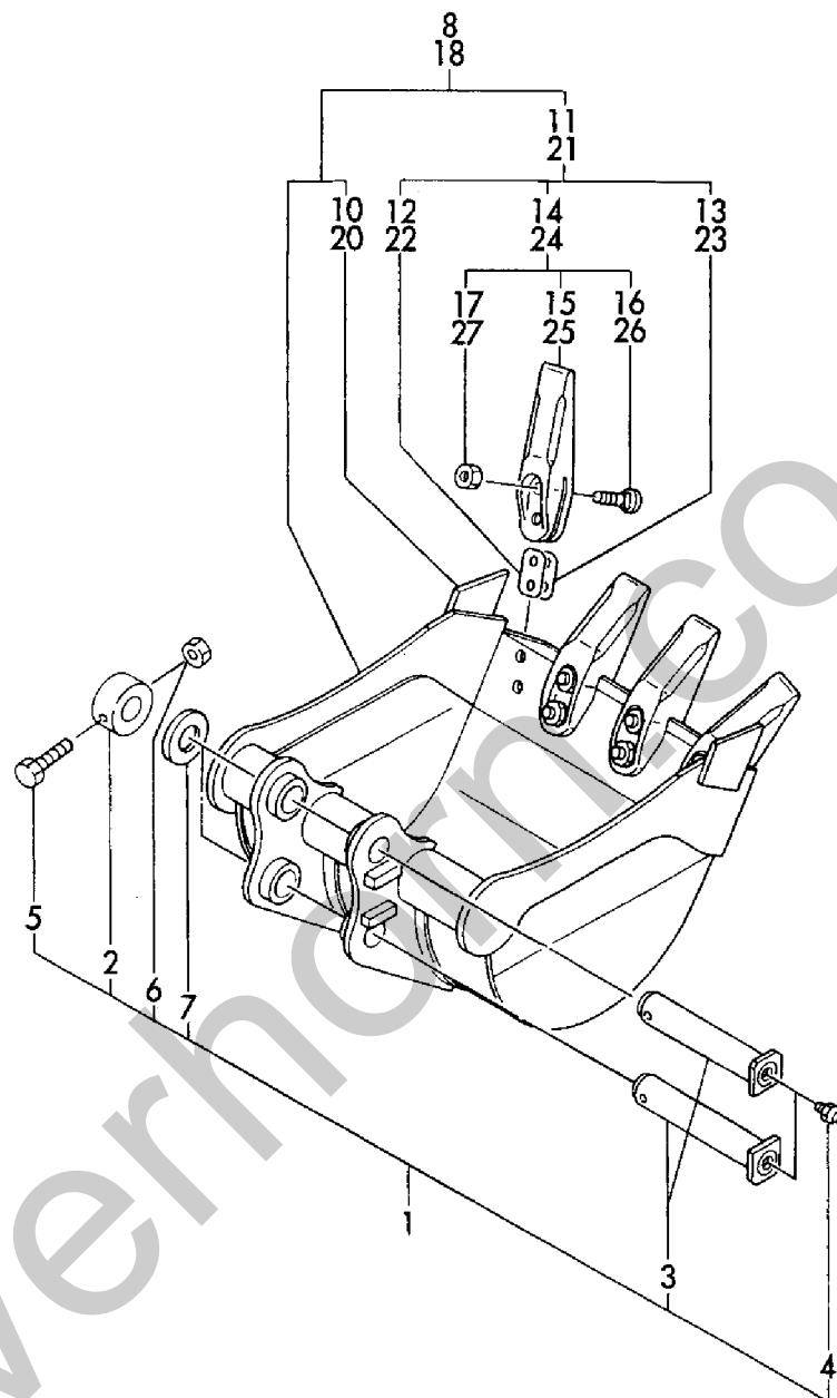
Fig. 59 バケット (400) (450) BUCKET (400) (450)
