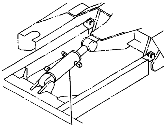
Fig. 36 ブレードシリンダ (B12/17-2) BLADE CYLINDER (B12/17-2)
