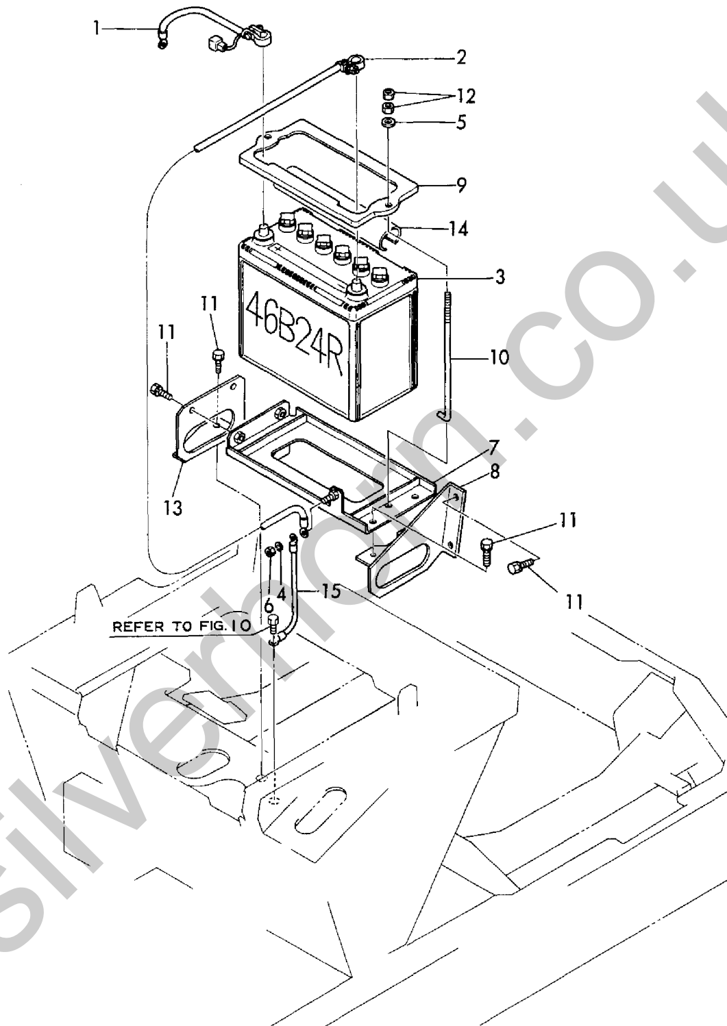
Fig. 9 バッテリー BATTERY
