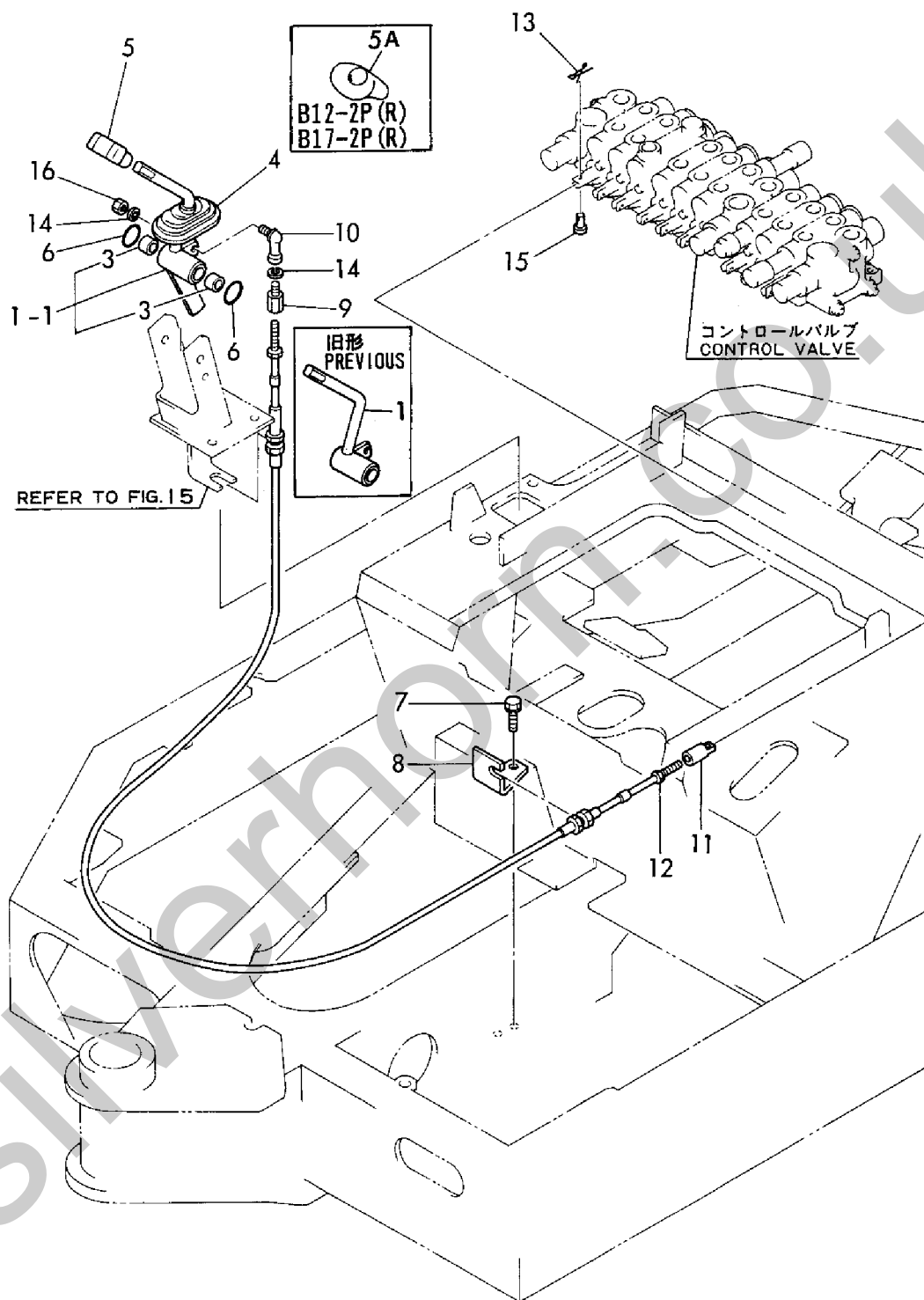
Fig. 19 操縦装置 (ブレード) CONTROL EQUIPMENT (BLADE)
