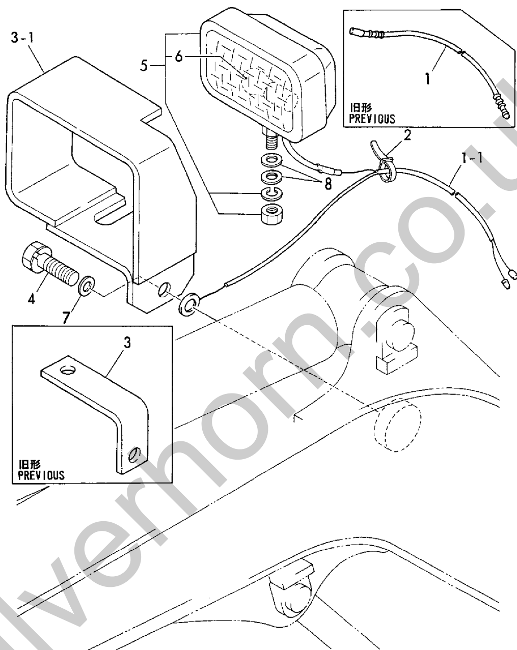
Fig. 11 ワークランプ WORK LAMP
